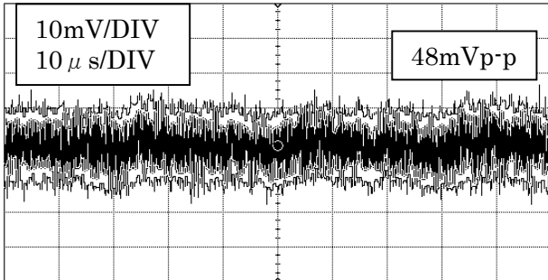
9V 入力, DC ジャック CN3A_1-2pin
