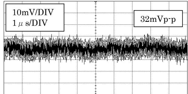
5V, ジャック, J4A_32pin
