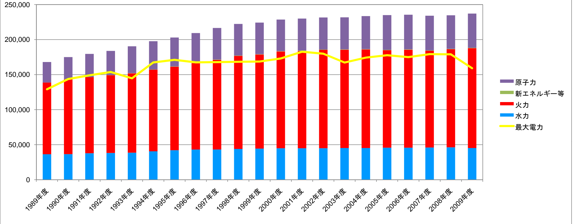
電気事業用最大出力と最大電力(全国) 単位：MW
