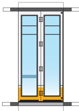
(前ドア)
